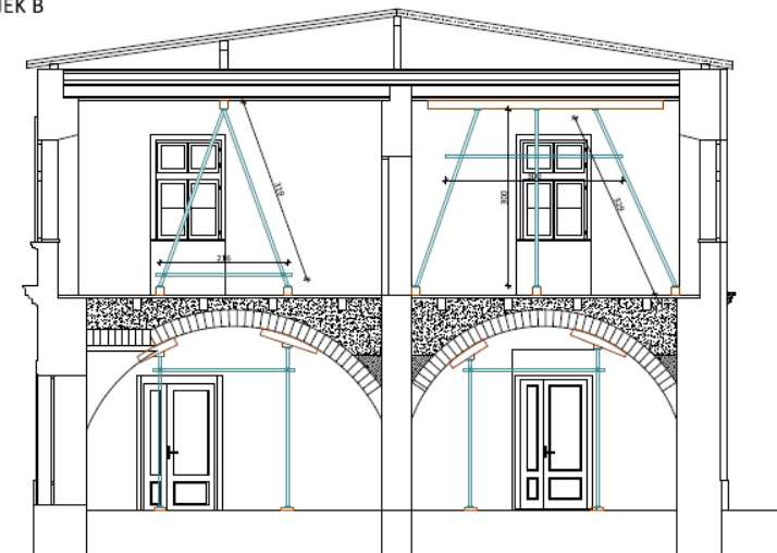
PRESJEK B
